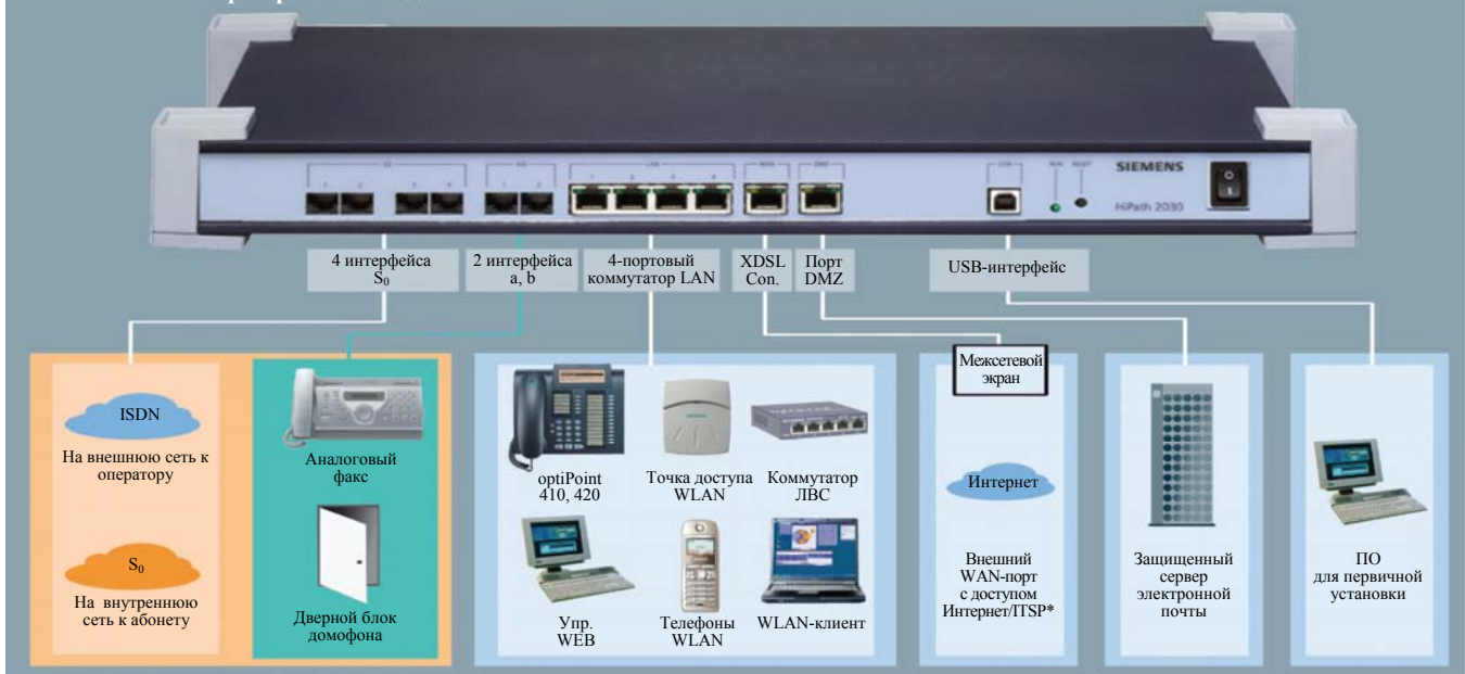
HiPath 2030 – обзор вариантов подключения
